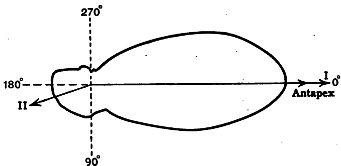
I. Region I. ; centre, North Pole.
